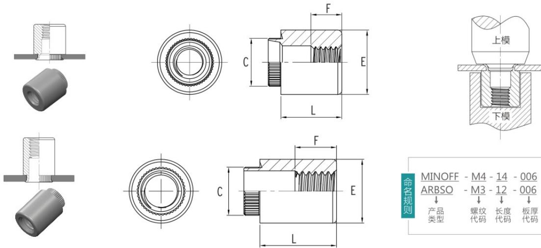
所有尺寸：毫米 通用尺寸数据表
